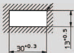
Schalttafelausschnitt
